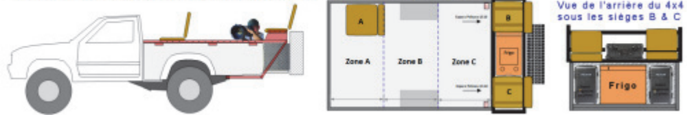
Représentation de la disposition modulable des sièges grâce à leur fixation par boulons et écrous et non pas soudés comme d'habitude. La totalité de la structure n'est pas représentée, notamment la protection par rapport au soleil. Les mesures et l'échelle sont indicatives.
